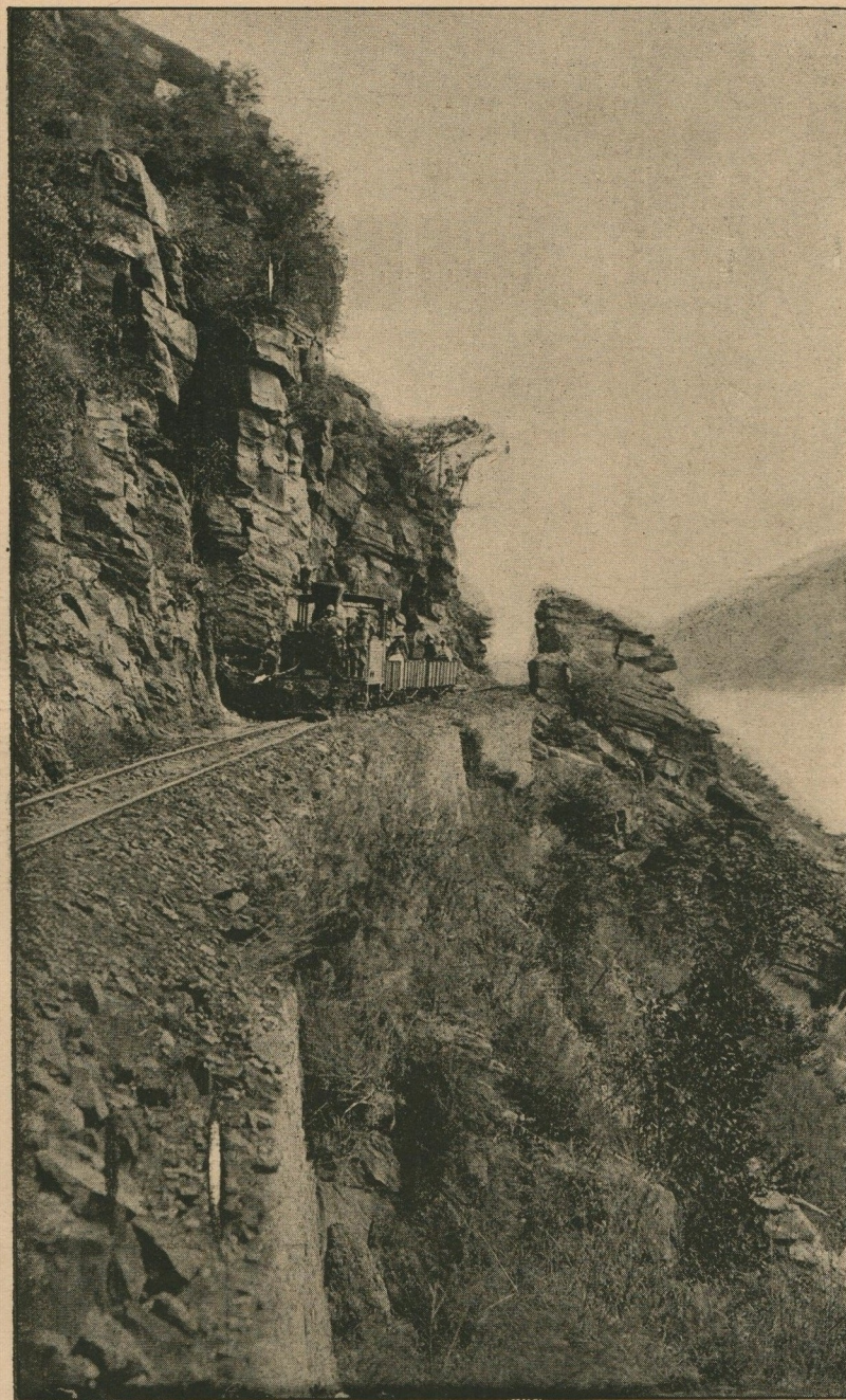
305. — Chemin de fer du Congo. La locomotive au kilomètre 2,700. Spoorweg van den Congo. De locomotief aan den kilometer 2,700.
